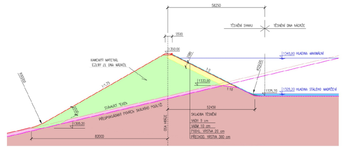
Horní nádrž - řez
