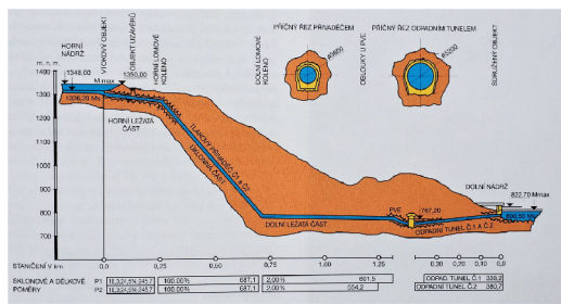
Hydraulický obvod PVE
