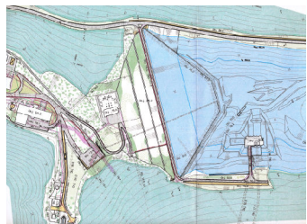
Dolní nádrž - situace
