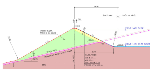
Dolní nádrž - řez
