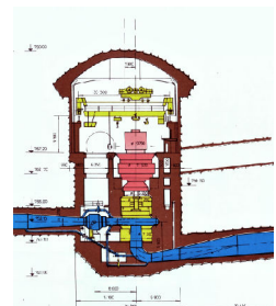
Příčný řez strojním blokem
