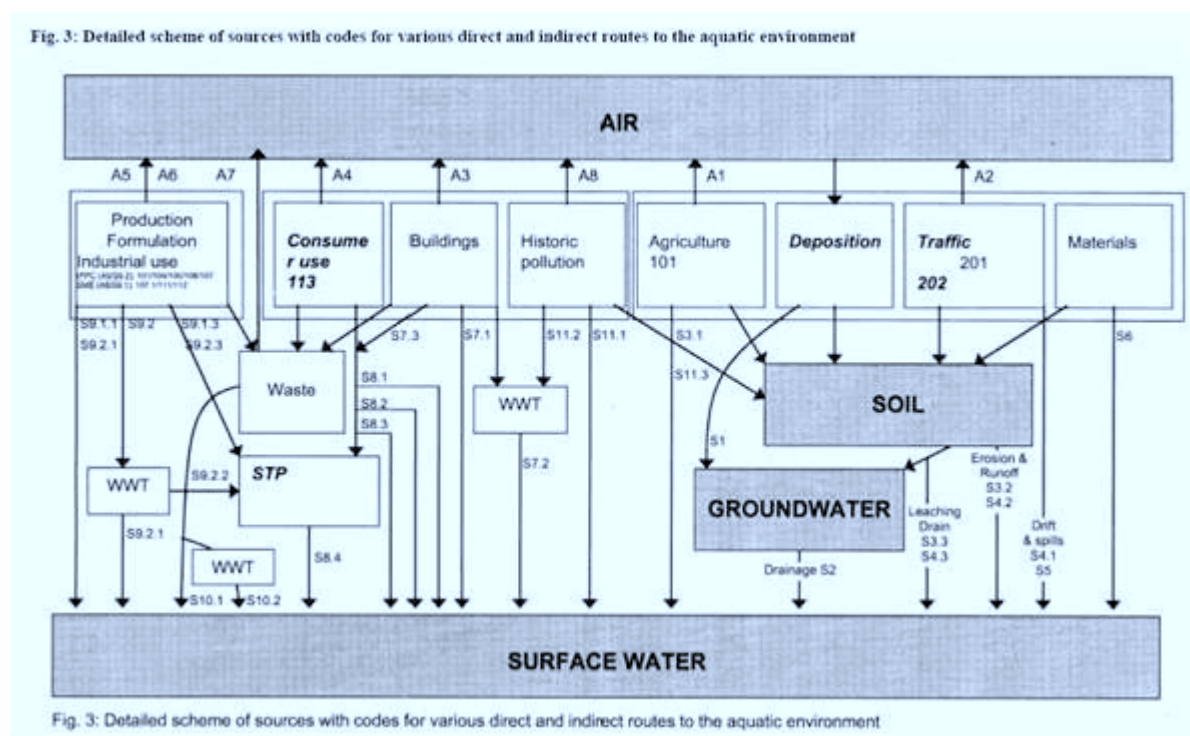
Obr. 2.5.1. Schéma zdrojů a cest znečišťujících látek (zdroj: Identification and Emission Controls, European Commission, 2006 )
