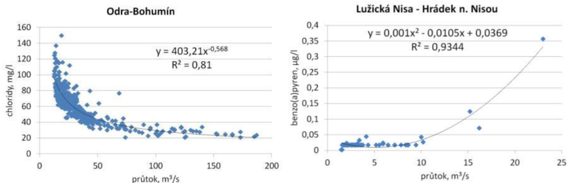
Obr. 2.10.7.1. Příklad závislosti koncentrace chloridů na průtoku (profil Odra-Bohumín, data z roku 1998, Povodí Odry, s.p.)
