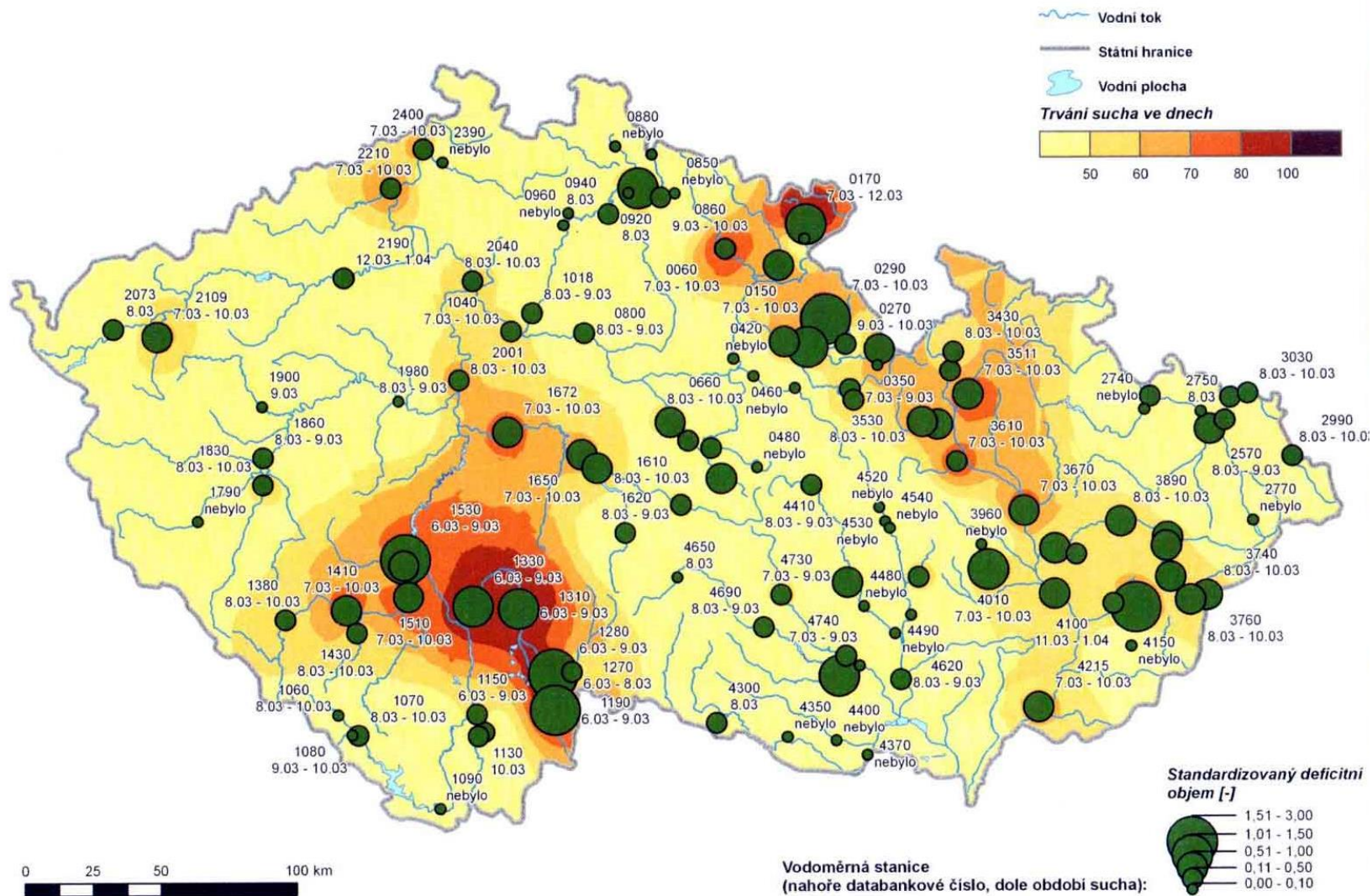
Obrázek 3.1-31 Mapa rozložení hydrologického sucha na území ČR v roce 2003. Limitem byl denní odtok překročený s 95% pravděpodobností v období 1961-2005.
