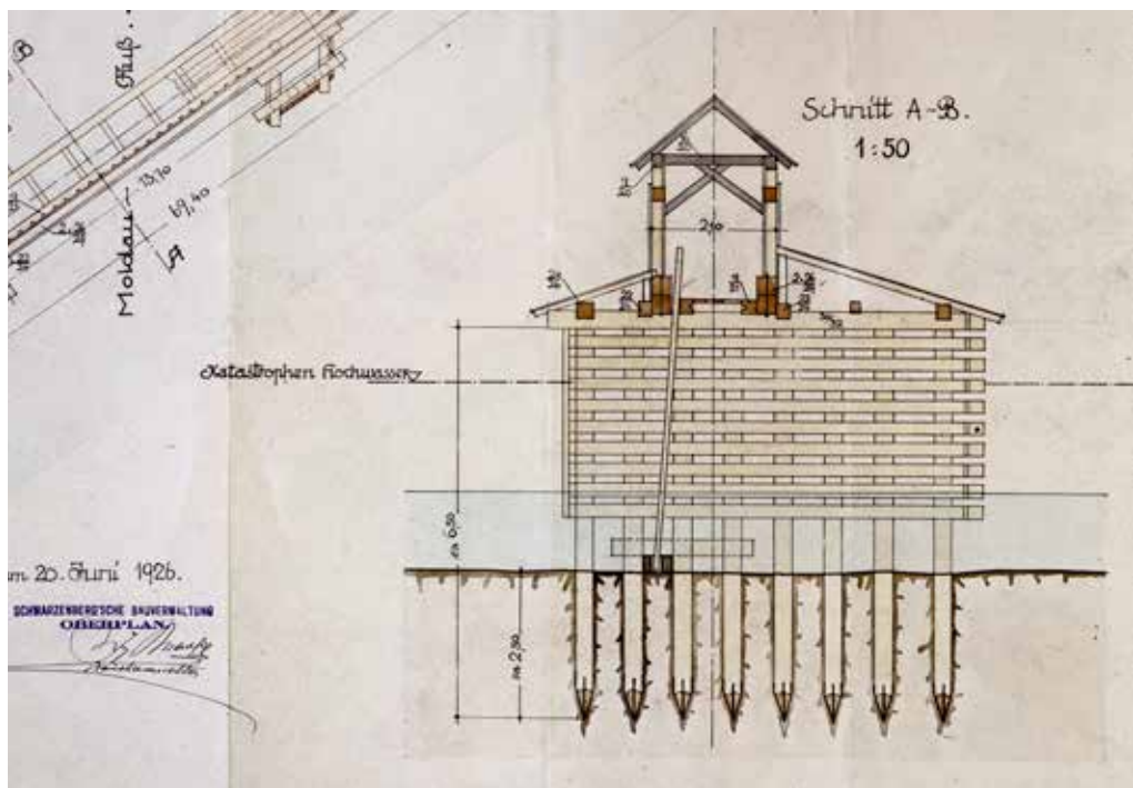
Obr. 19. Plán na opravu rechlí nazývaných Spitzenberg (Hory), Markl, 1926, řez, zdroj: SOA v Třeboni, odd. Český Krumlov, fond Schwarzenberská ústřední stavební správa České Budějovice, plán č. 3147
