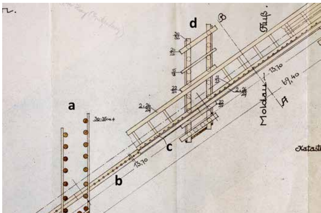
Obr. 18. Plán na opravu rechlí nazývaných Spitzenberg (Hory), Markl, 1926, detail půdorysu, zdroj: SOA v Třeboni, odd. Český Krumlov, fond Schwarzenberská ústřední stavební správa České Budějovice, plán č. 3147. Legenda: a – založení dvouráde mostní básky v úrovni říčního dna; b – prahové trámký ve dně řeky pro aretaci tyčí brlení; c – trám s dlabý pro vložení tyčí brlení v úrovni lávky, před ním dobře patrná mezera pro manipulaci s brlením při jeho instalaci a vyjímání; d – zpevnění básky klešinami a fošnami pod lávkou
