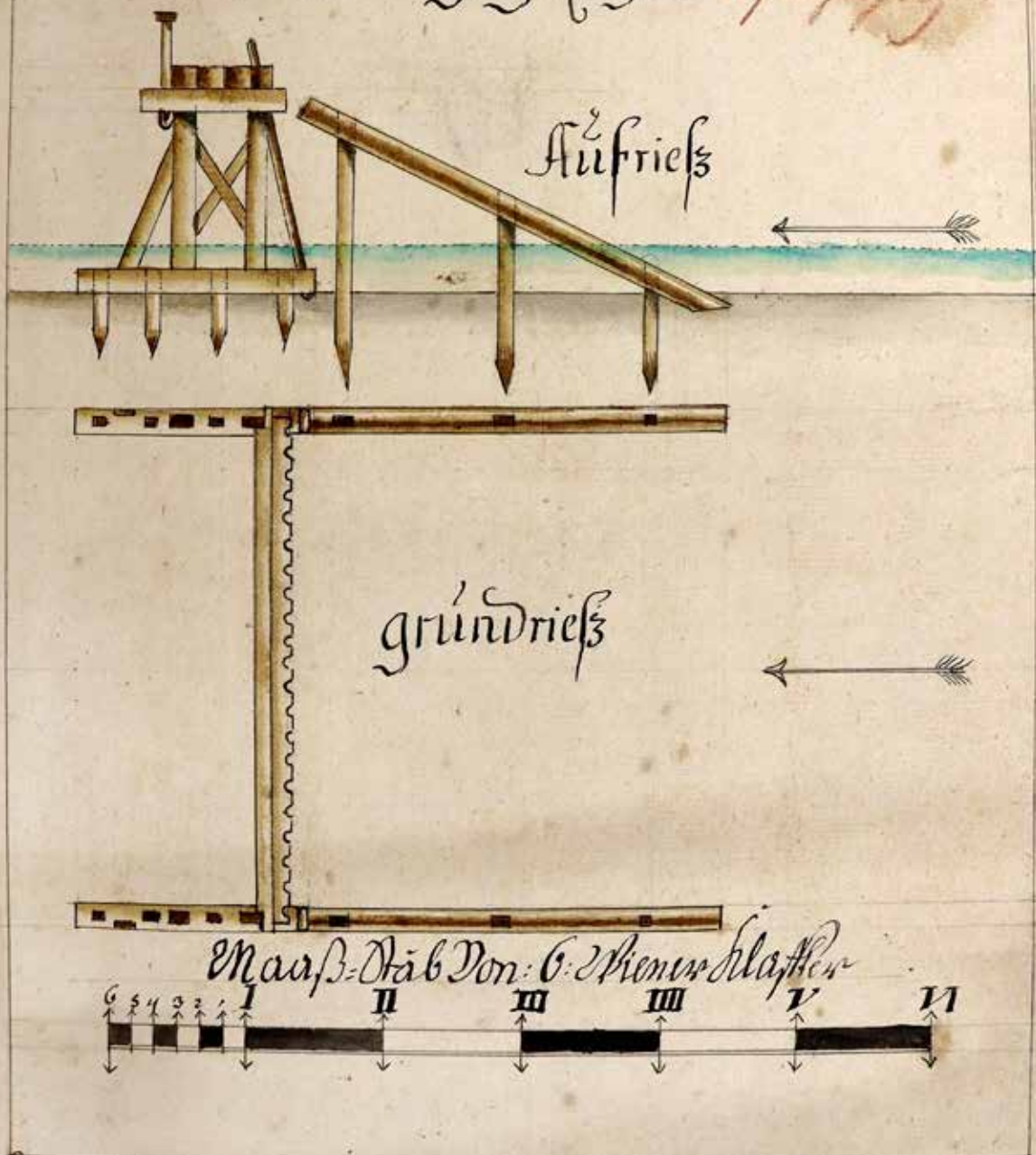
Obr. 26. Plán rechlí nazývaných Ponholz nedaleko Blanska u Kaplice, Johan Franz Riemer, 1780, zdroj: SOA v Třeboni, odd. Třeboň, fond Vs Nové Hradý, oddíl voroplavba
