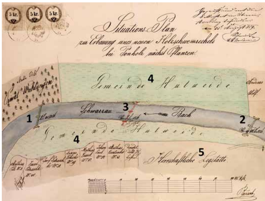
Obr. 28. Situační plán k výstavbě nových rechlí Ponholz nedaleko Blanska u Kaplice, 1859, zdroj: SOKA Český Krumlov, fond OÚ Kaplice, kart. č. 10. Legenda: 1 – umístění rechlí postavených roku 1780/1781, na místě do roku 1806; 2 – umístění rechlí postavených roku 1806, na místě do roku 1836; 3 – umístění dřevěných rechlí postavených roku 1836, roku 1859/1860 nahrazených novými na kamenných pilířích; 4 – obecní pastviny; 5 – vrchnostenské skladiště dřeva
