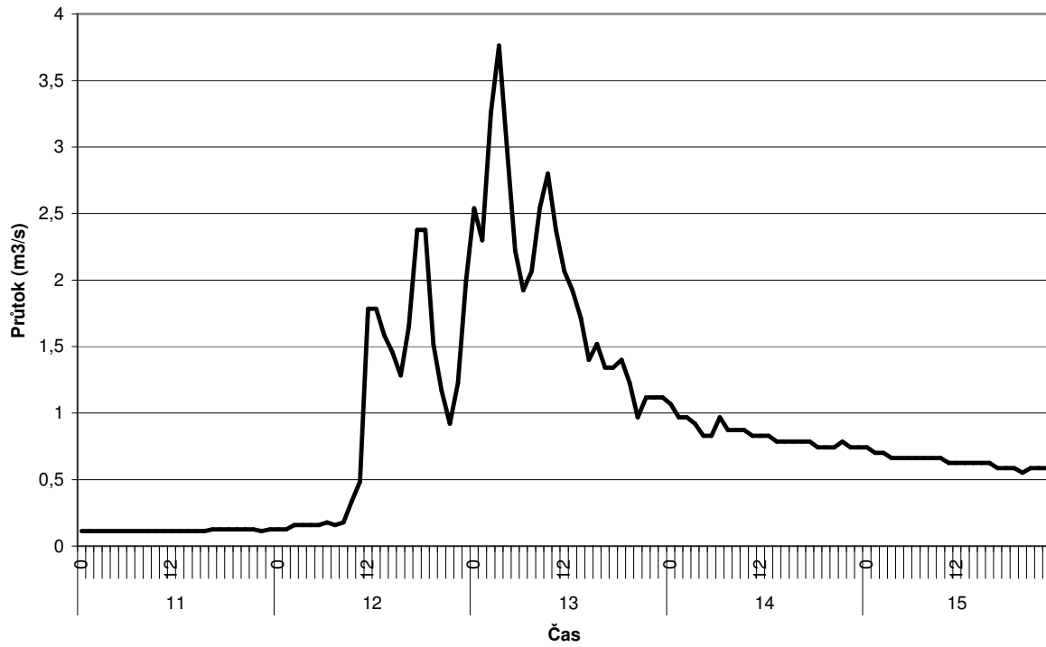
Obr.4 Hydrogram průtoku - Hutná nad štěrkovou přepážkou Málkov, srpen 2002
