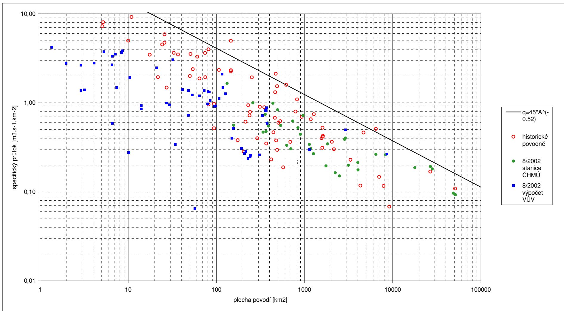
Obr. 5 Specifické kulminační průtoky k plochám povodí
